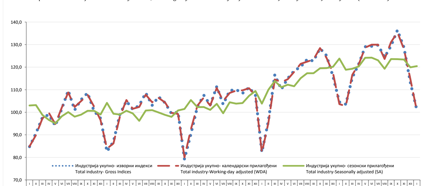
График 1. Временска серија индустрија укупно - изворни, календарски и сезонски прилагођени индекси: јануар 2014 - јануар 2019 (2015 = 100) Graph 1. Time series for total industry - Gross, Working-day and Seasonally Adjusted indices: January 2014 - January 2019(2015=100)
