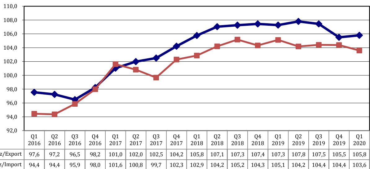
Indeksi jediničnih vrijednosti izvoza i uvoza, po tromjesečjima 2016.-2020. godine (KM) Unit value indices of export and import, by quarters 2016-2020 (KM)
