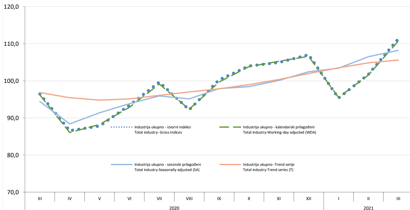
Grafik 1. Mjesečna serija indeksa industrija ukupno - izvorni, kalendarski i sezonski prilagođeni indeksi: ožujak 2020. - ožujak 2021. (2015=100) Graph 1. Monthly series of industrial indices for total - Gross, Working-day and Seasonally Adjusted indices: March 2020 - March 2021 (2015=100)
