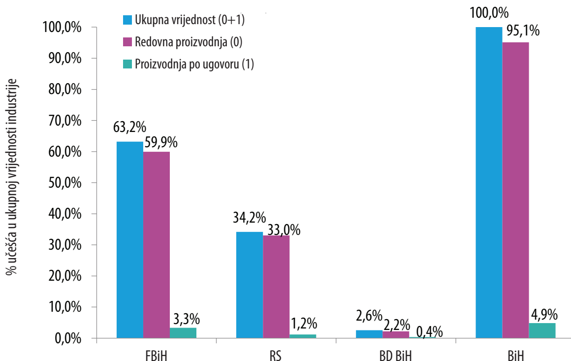
Grafikon 4. Struktura vrijednosti prodaje/isporuke industrijskih proizvoda u 2023. godini po vrsti proizvodnje i entitetima
