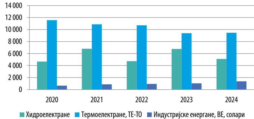
Бруто производња електричне енергије
