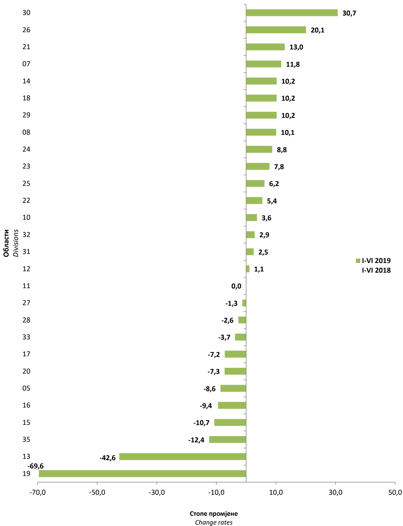
График 4. Годишње стопе промјене индустријске производње из календарски прилагођених индекса, I - VI 2019 / I - VI 2018
