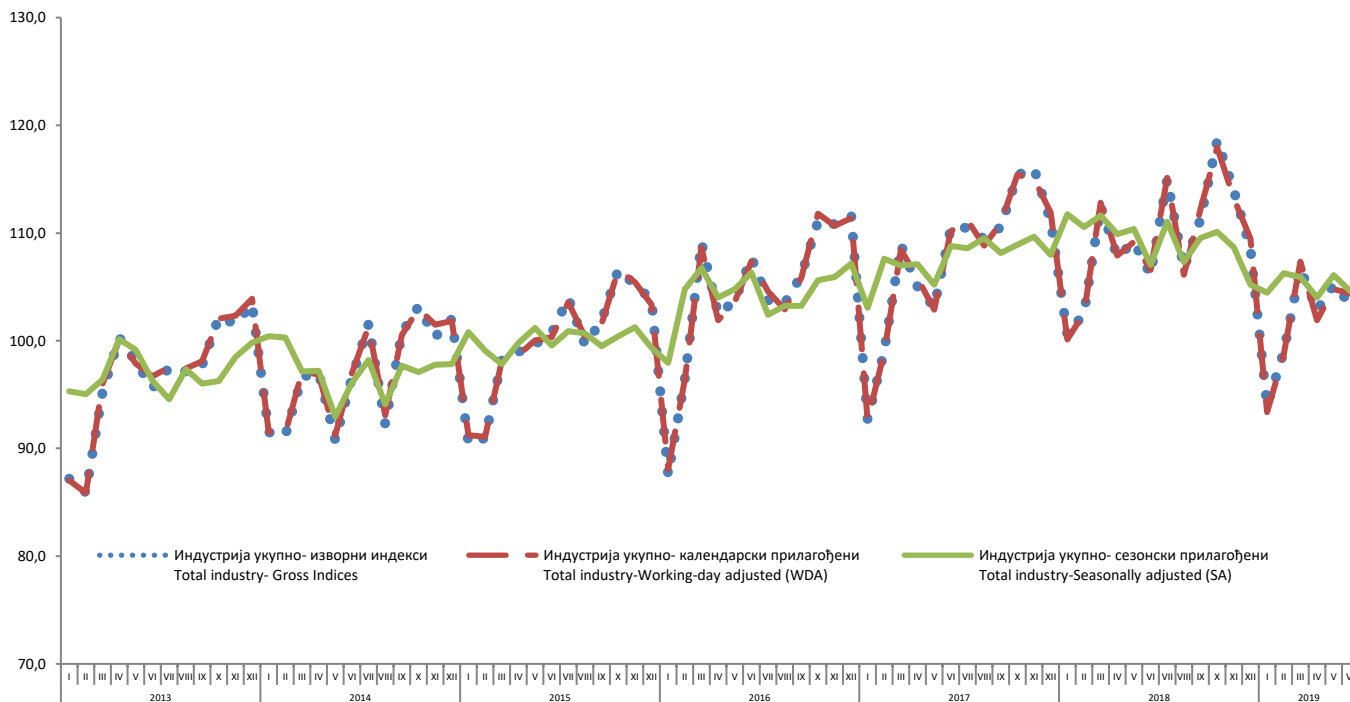
График 1. Временска серија индустрија укупно - изворни, календарски и сезонски прилагођени индекси: јануар 2013 - јун 2019 (2015 = 100) Graph 1. Time series for total industry - Gross, Working-day and Seasonally Adjusted indices: January 2013 - June 2019 (2015=100)
