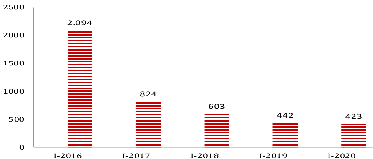
Г.6. Превезени терет у ваздушном саобраћају, тона G.6. Transported cargo air traffic, tons
