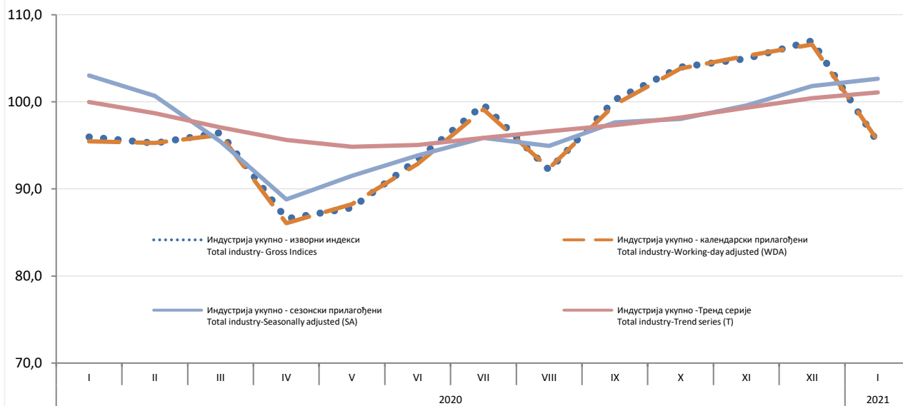
График 1. Мјесечна серија индекса индустрија укупно - изворни, календарски и сезонски прилагођени индекси: јануар 2020 - јануар 2021 (2015 = 100) Graph 1. Monthly series of industrial indices for total - Gross, Working-day and Seasonally Adjusted indices: January 2020 - January 2021 (2015=100)
