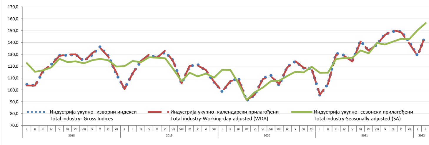
График 1. Временска серија индустрија укупно - изворни, календарски и сезонски прилагођени индекси: јануар 2018 - фебруар 2022 (2015 = 100) Graph 1. Time series for total industry - Gross, Working-day and Seasonally Adjusted indices: January 2018 - February 2022 (2015=100)
