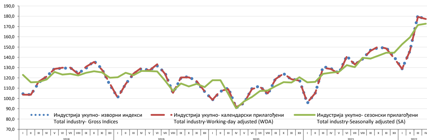
График 1. Временска серија индустрија укупно - изворни, календарски и сезонски прилагођени индекси: јануар 2018 - април 2022 (2015 = 100) Graph 1. Time series for total industry - Gross, Working-day and Seasonally Adjusted indices: January 2018 - April 2022 (2015=100)
