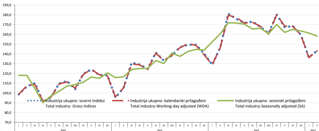
Grafik 1. Vremenska serija industrija ukupno - izvorni, kalendarski i sezonski prilagođeni indeksi: januar 2020 - februar 2023 (2015=100) Graph 1. Time series for total industry - Gross, Working-day and Seasonally Adjusted indices: January 2020 - February 2023 (2015=100)
