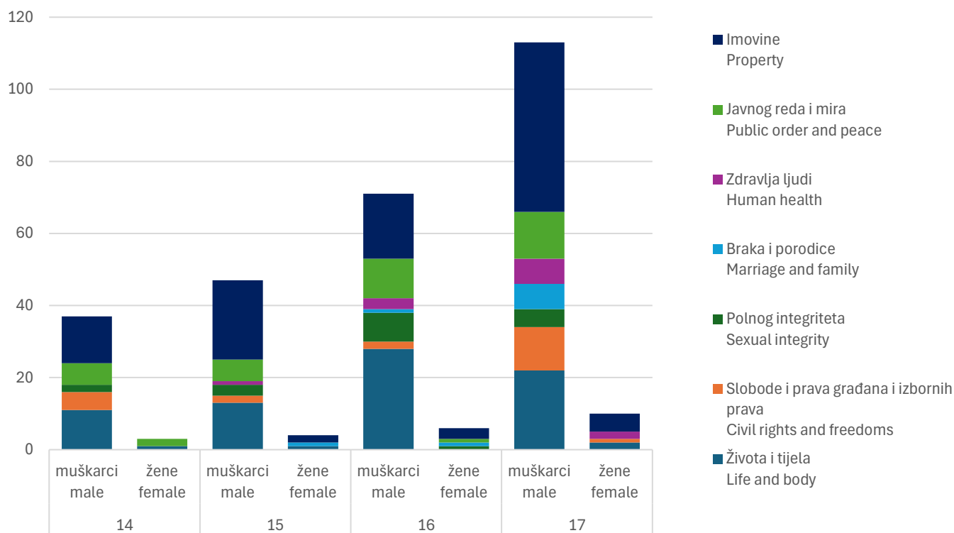
Grafikon 2. Prijavljene maloljetne osobe prema skupinama kaznenih djela i starosti Graph 2 Reported juvenile offenders by types of criminal offenses and age
