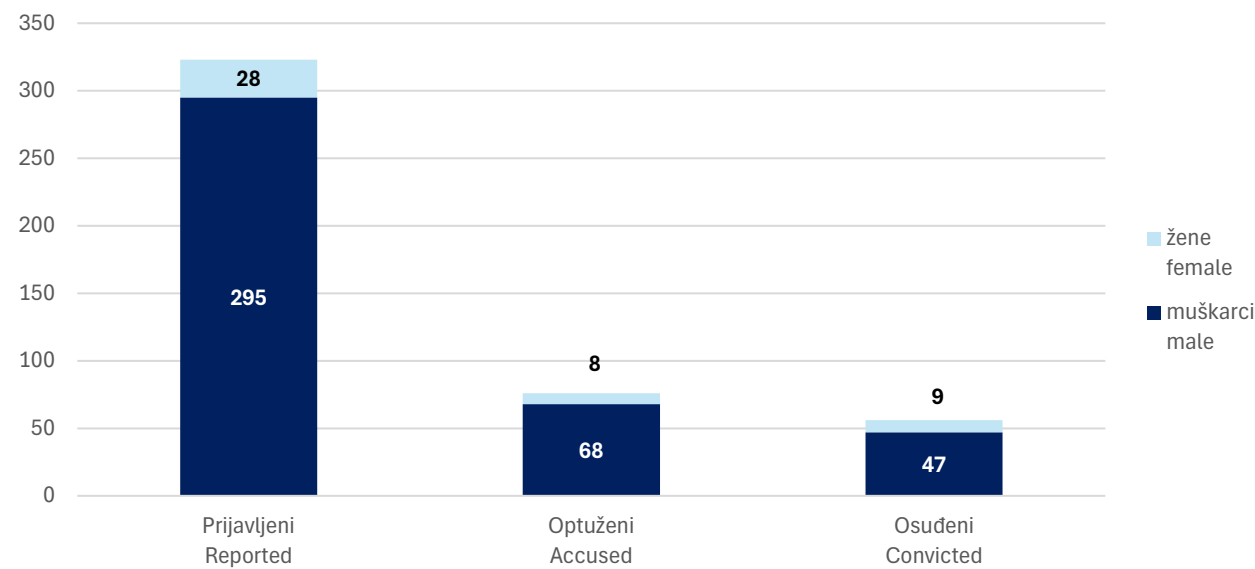
Grafikon 1. Maloljetni učinitelji kaznenih djela u BiH – prijavljeni, optuženi i osuđeni, 2024. Graph 1. Juvenile perpetrators of criminal offences in BiH- reported, accused and convicted, year 2024
