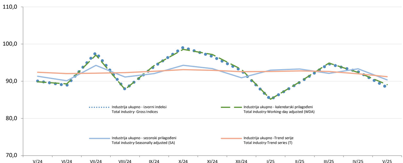
Grafikon 1. Mjesečna serija indeksa industrija ukupno - izvorni, kolendarski i sezonski prilagođeni indeksi: svibanj 2024. - svibanj 2025. (2021=100) Graph 1. Monthly series of industrial indices for total - Gross, Working-day and Seasonally Adjusted indices: May 2024 - May 2025 (2021=100)
