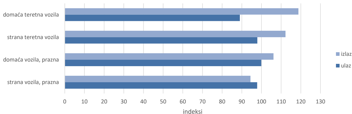
Grafikon 1: Cestovni granični promet teretnih motornih vozila, I tromjesečje 2025./ I tromjesečje 2024.
